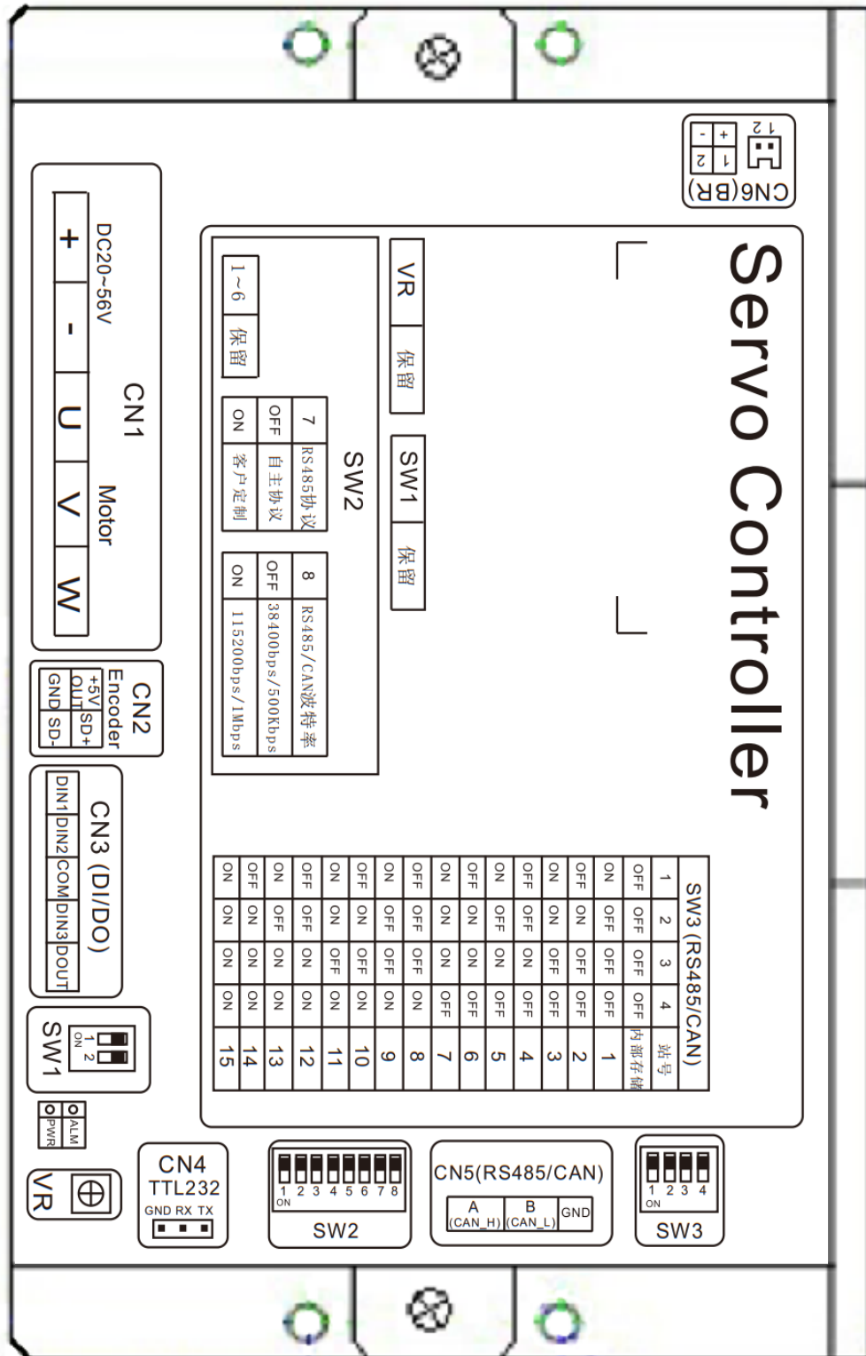
4.1.1 外壳丝印
